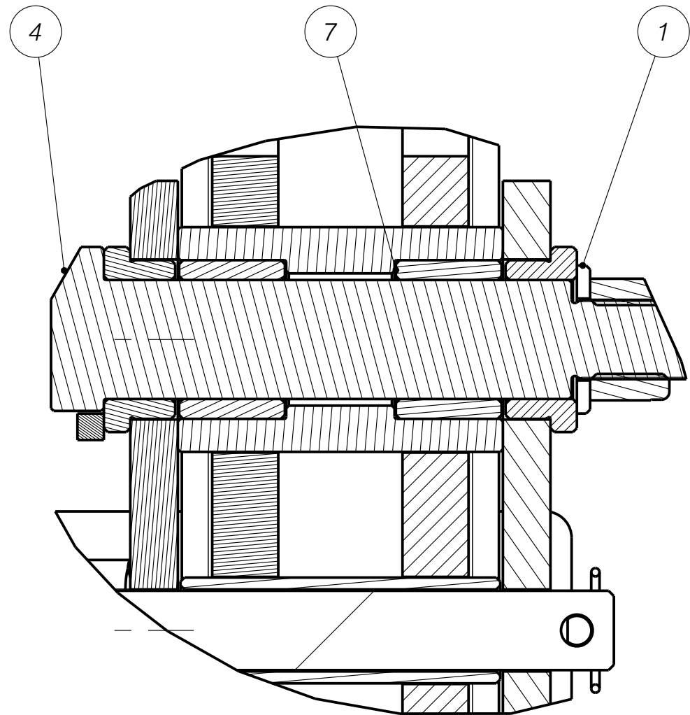
DETALLE A MONTAJE CASQUILLOS ESCALA 1:2
