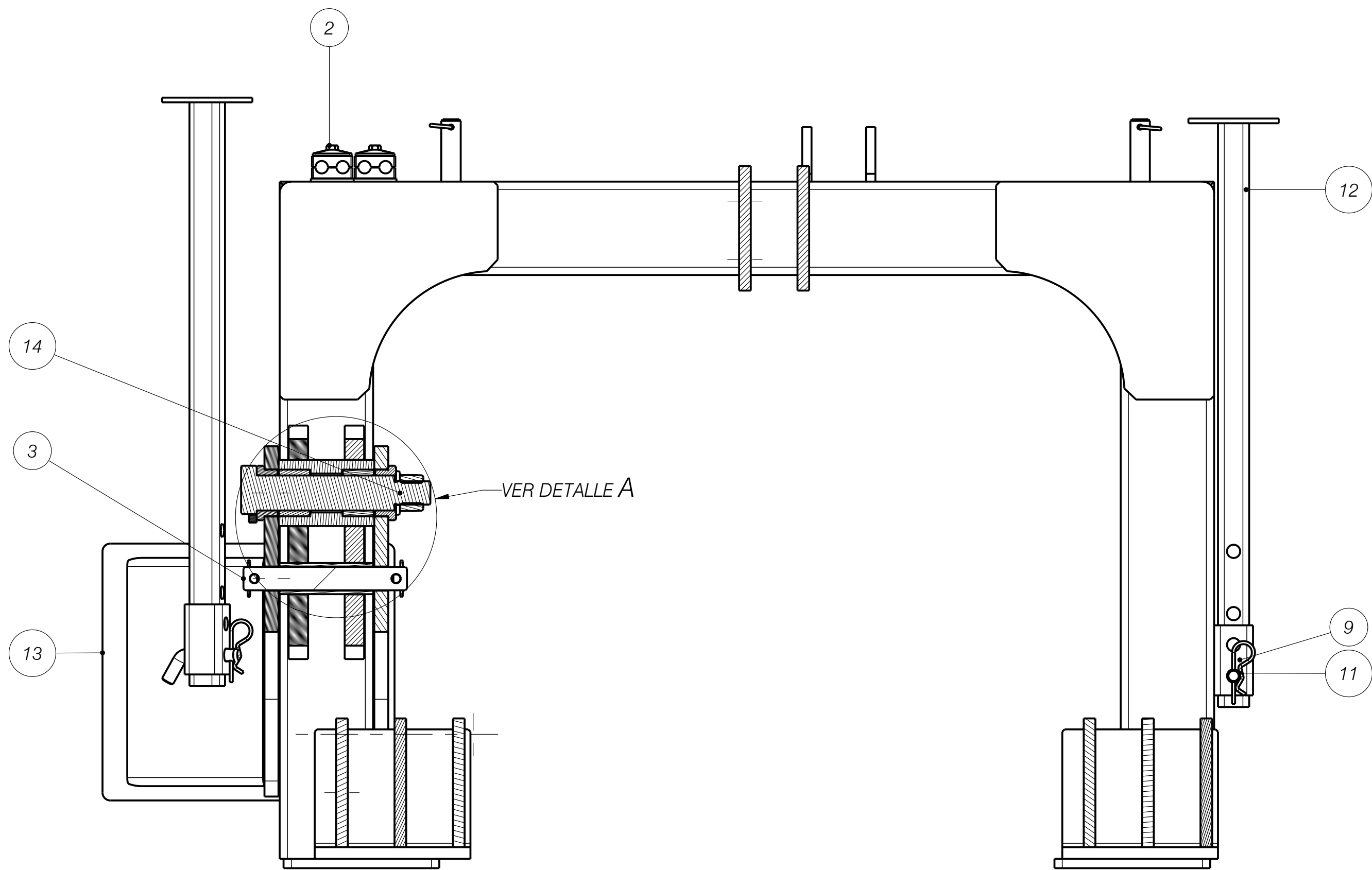
SECCIÓN A-A
